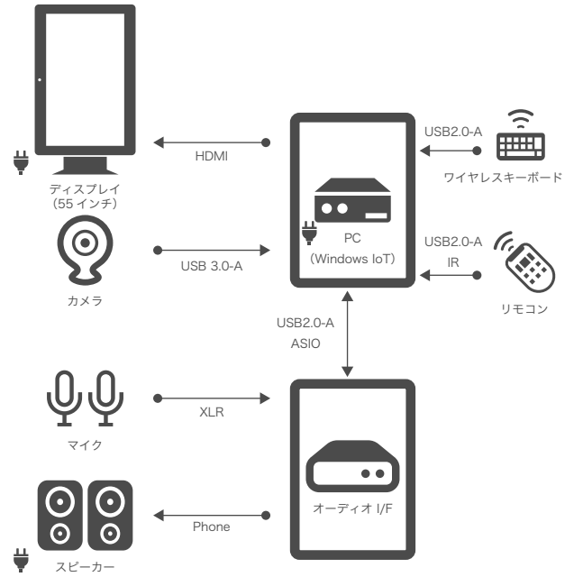
結線図
